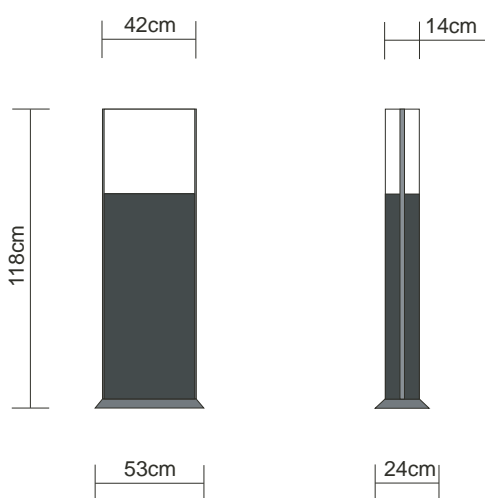
Ansicht Front
